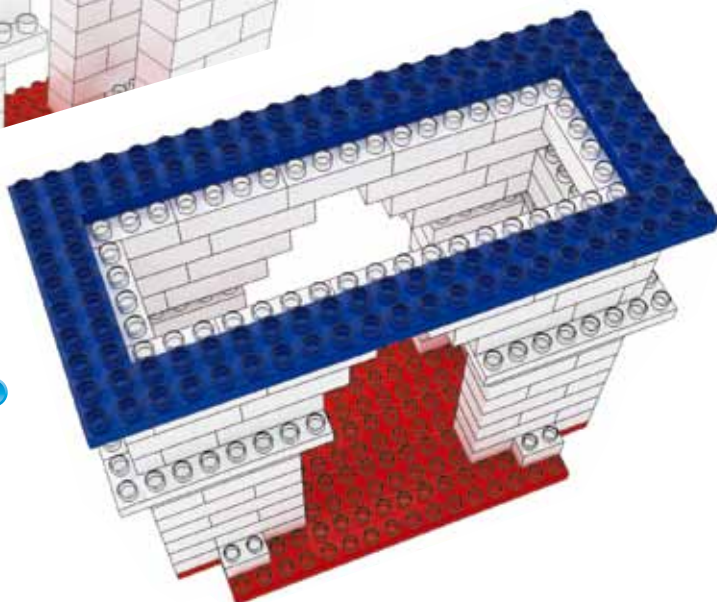
Fig. | 9 Armado segunda saliente
