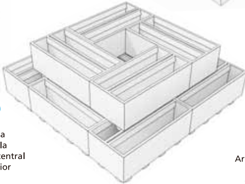
Fig. | 9 Armado parte inferior de columna central
