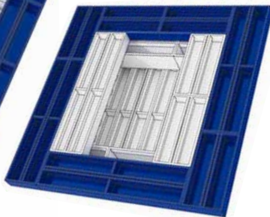
Fig. | 21 Montado traba de ventanas
