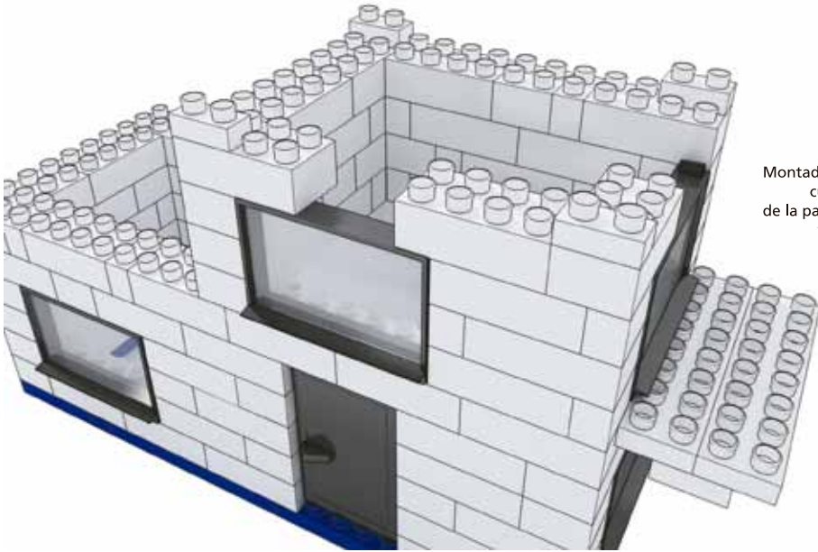
Fig. | 20 Montado parcial de cuarta hilada de la parte superior vista trasera
