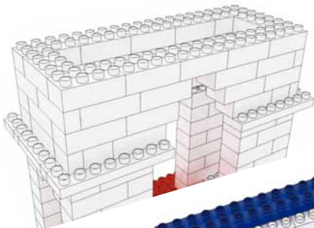
Fig. | 8 Arco superior terminado
