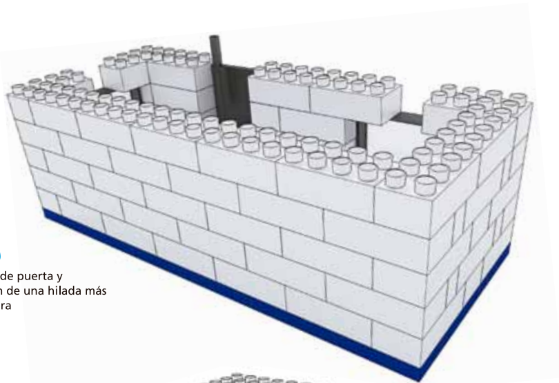
Fig. | 8 Ultima hilada de la parte inferior de la casa vista frontal
